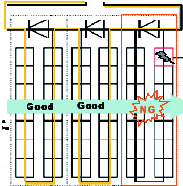
[태양전지 모듈 회로 구성]
